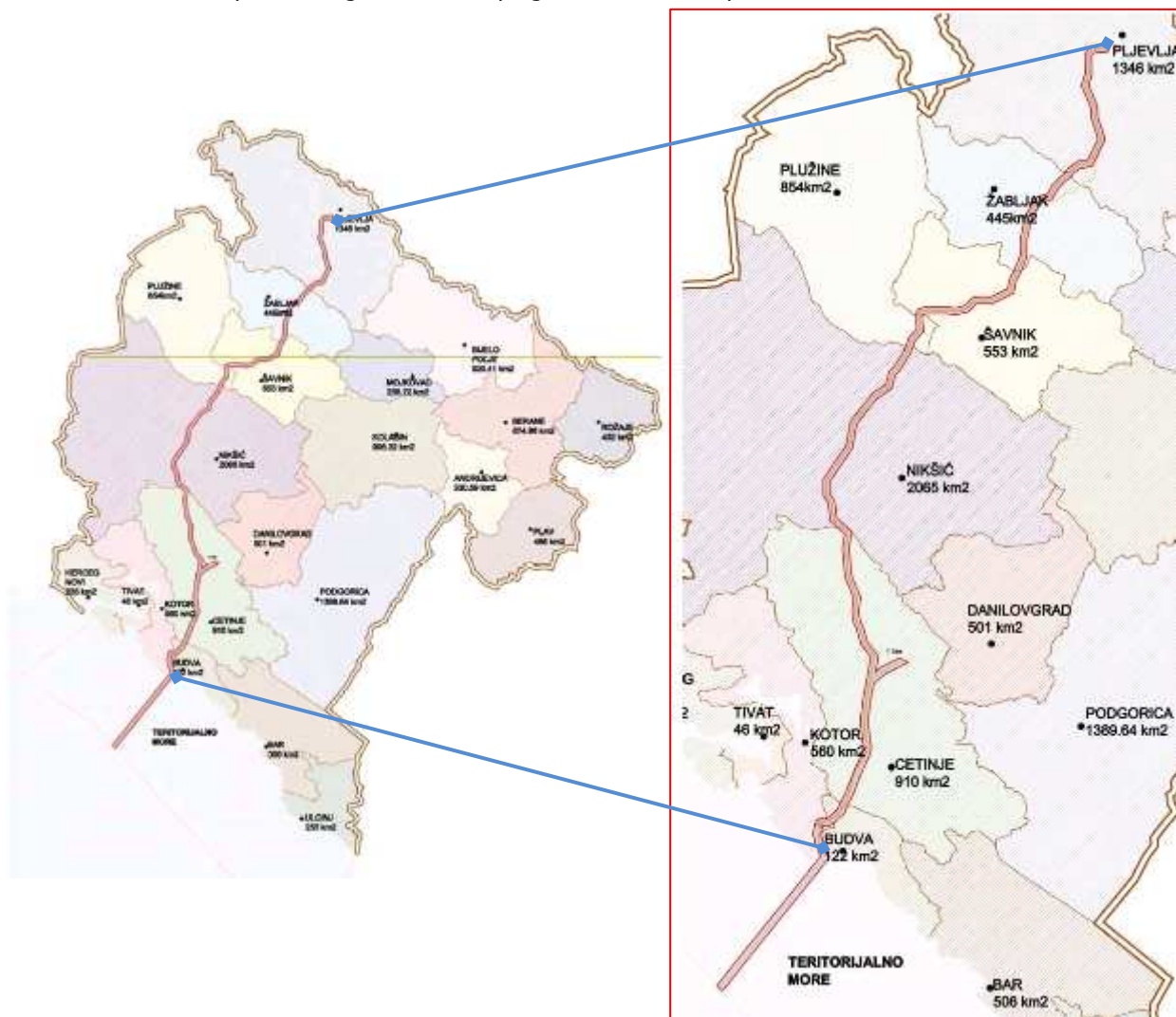
Slika 1 – trasa predloženog dalekovoda i pregled obuhvaćenih opština
