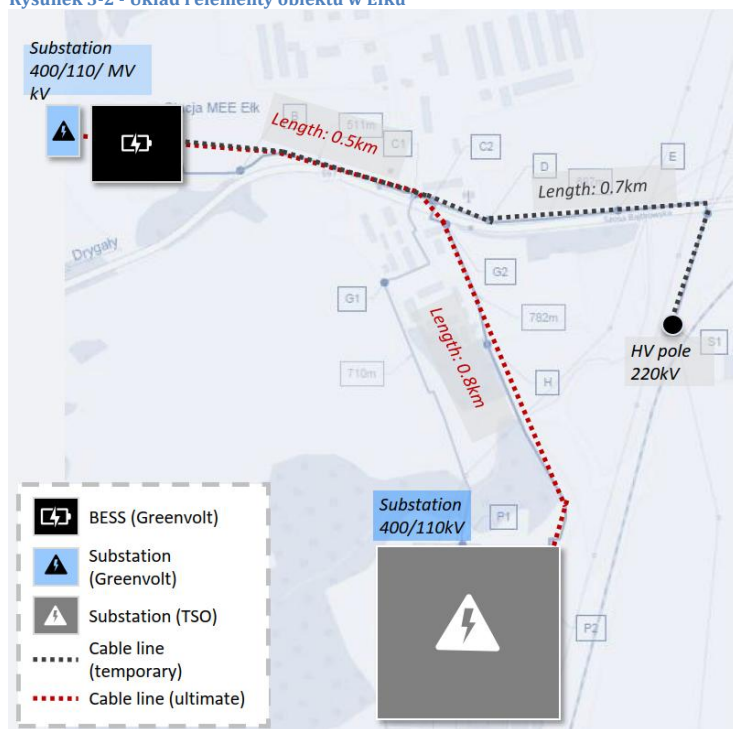
Rysunek 3-2 - Układ i elementy obiektu w Elku
