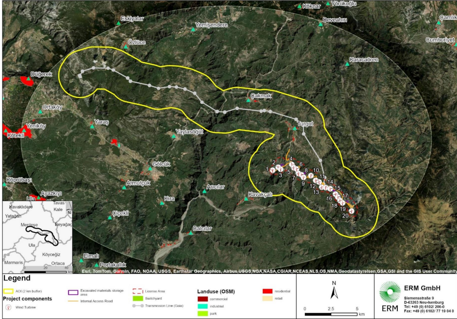
ŞEKİL 2-2 PROJE YERLEŞİM PLANI -1
