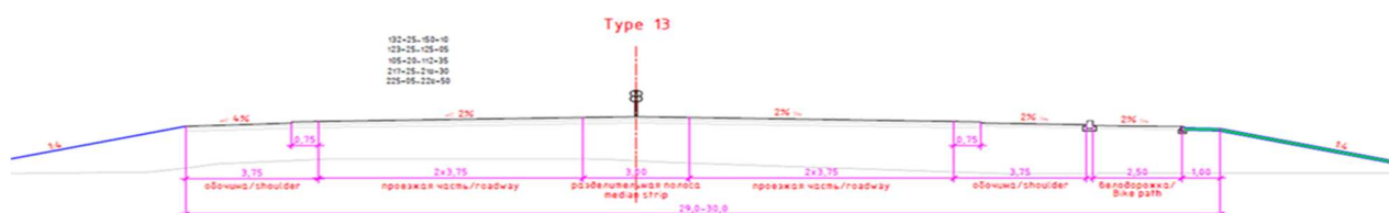
Расми 1 - Шакли муқаррари типӣ берун аз маҳалли аҳолинишин (4 хати роҳ. Категорияи техникии I)
